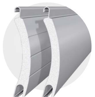
Aluminiumprofil A53 optional in glatter Optik
